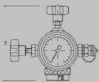
Urządzenia napełniające azotem
